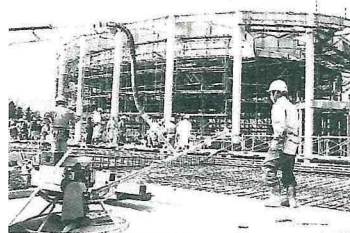
▼レールプレート敷設工事
