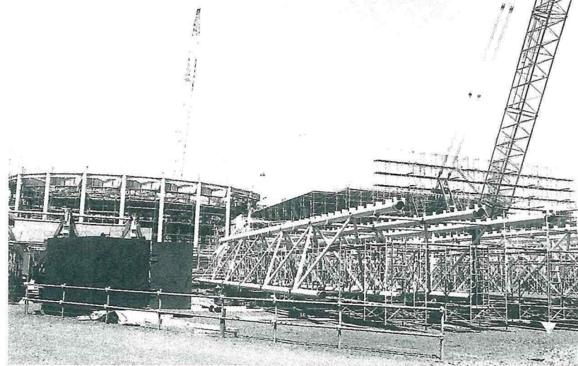
▲屋根大架構鉄骨が林立する現場。
