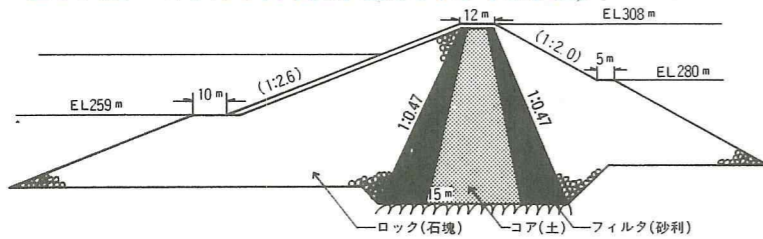
■七ヶ宿ダムのかたち(中央コア型ロックフィルダム)
