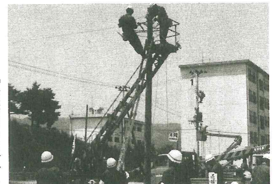
▲ 電話・電力施設の応急復旧訓練
