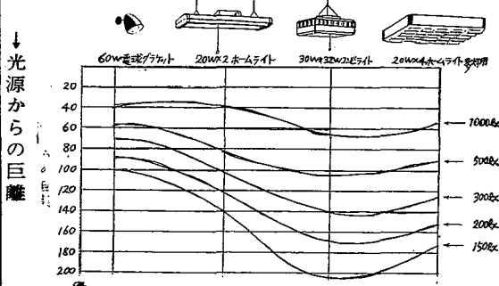
各種照明器具による照度
