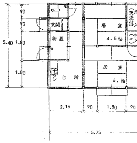
第二種 木造住宅平面図 建坪 31.05㎡ (9.5坪)
