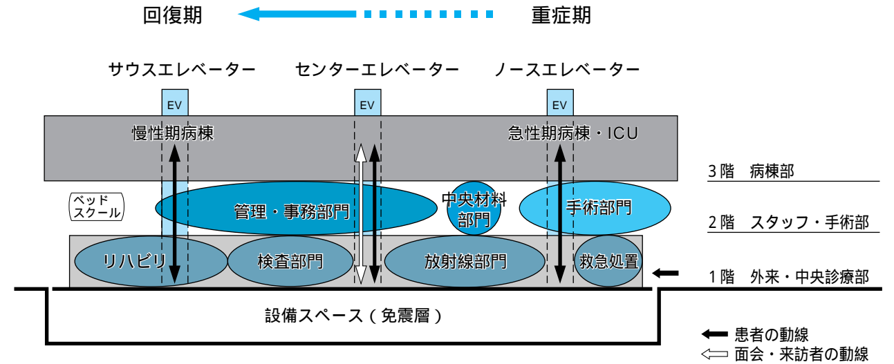
断面構成説明図
