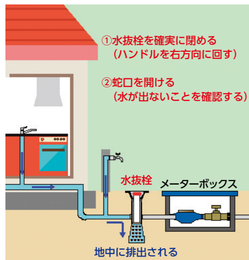
▲水抜きの操作手順
